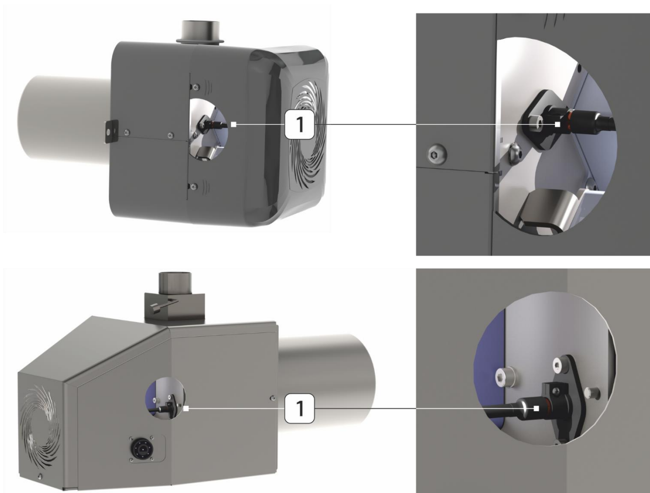
Rys. 12. Pozycja fotosensora w palniku REVO.
