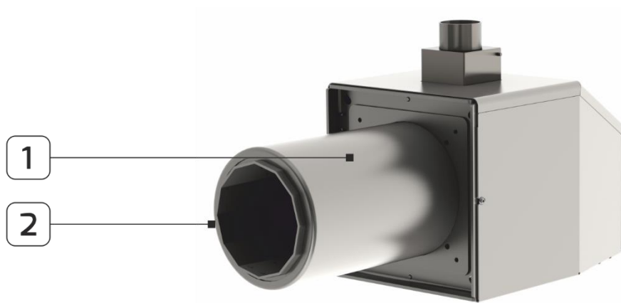
Rys. 11. Konserwacja REVO 44 do REVO 150.
