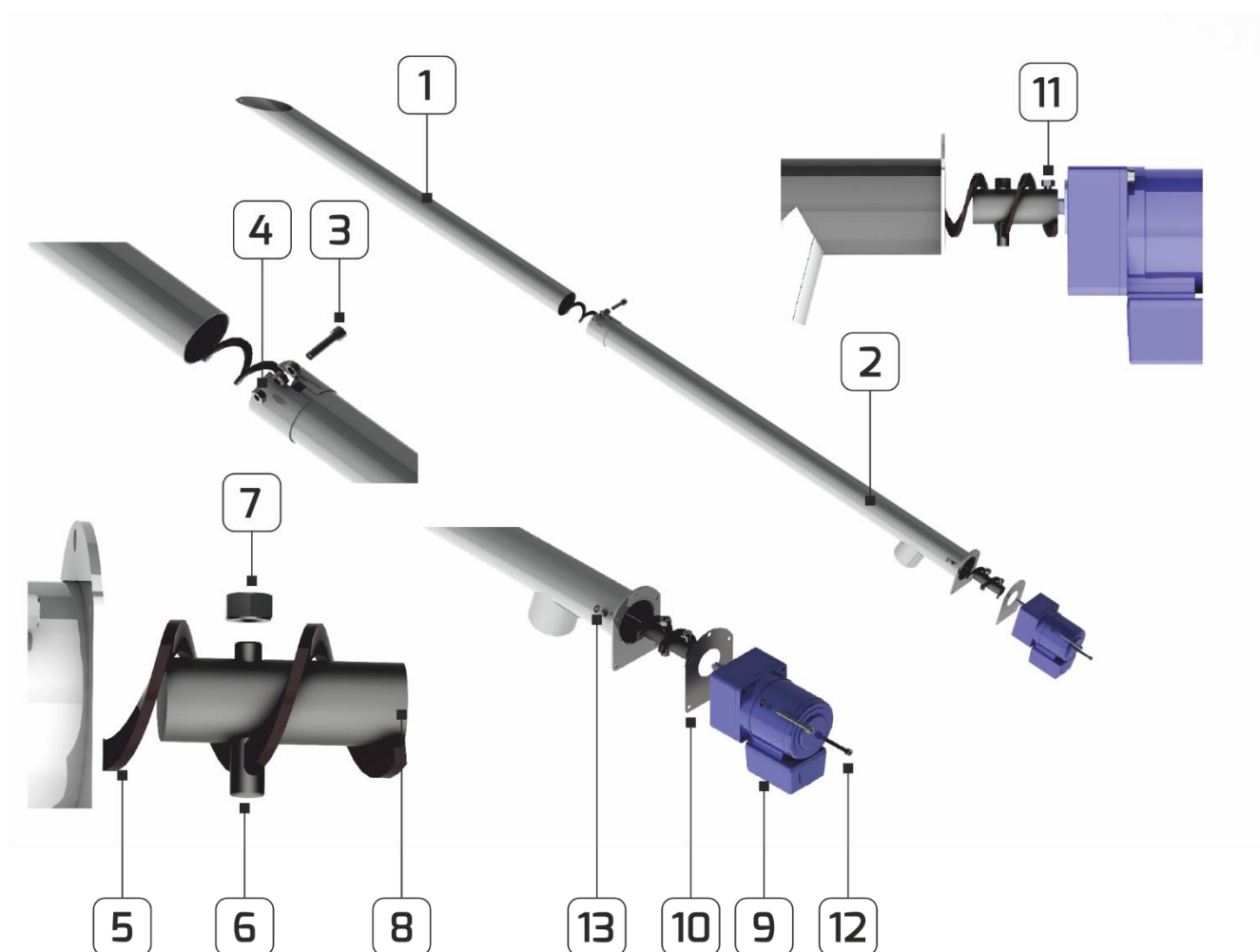
Rys.5. Budowa podajnika.
