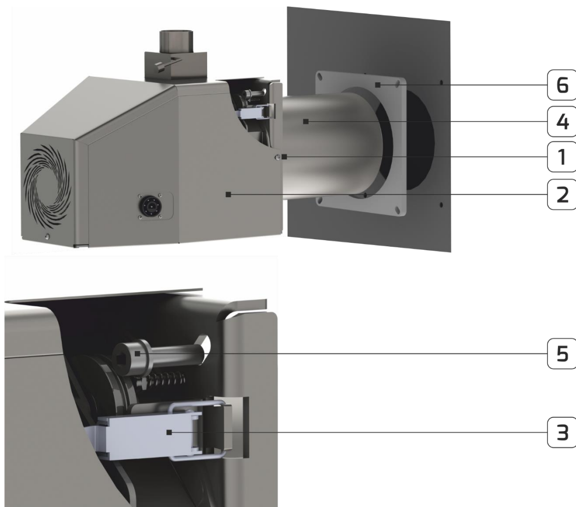
Rys. 9 Montaż modeli REVO 44 do REVO 150 w drzwiczkach kotła.
