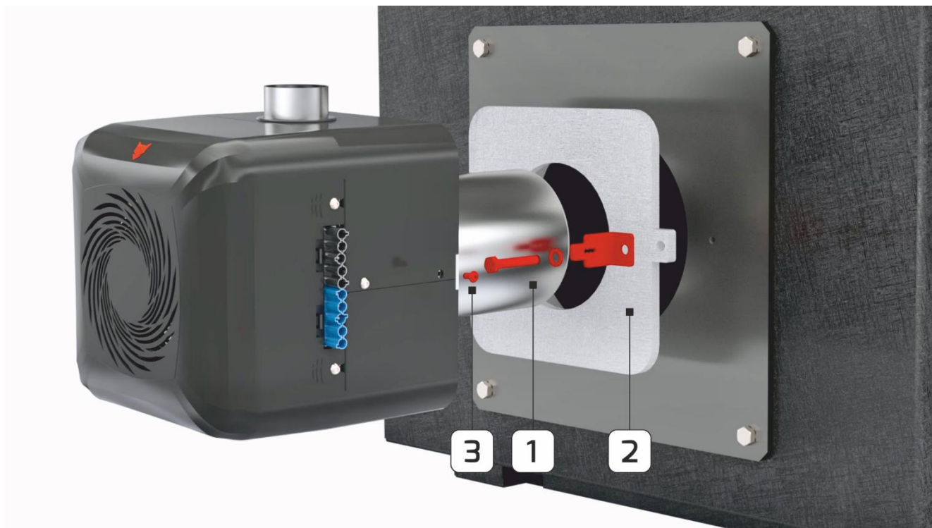
Rys. 8. Montaż palnika REVO Mini i REVO Mini 35.
