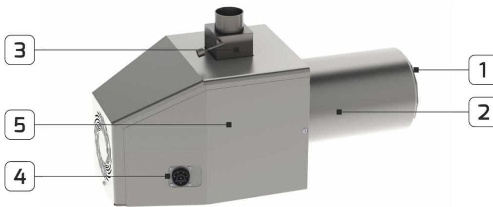
Rys. 2. Budowa palnika REVO 44 do REVO 150.
